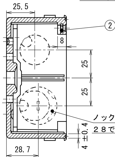
A-A 断面図
